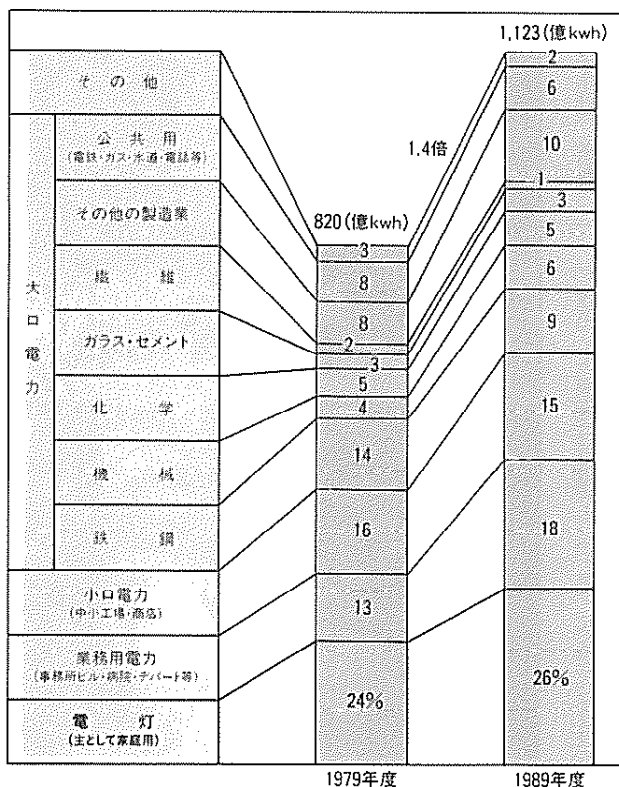
暮らしの中の電気(関西電力の場合) 販売電力量の推移
