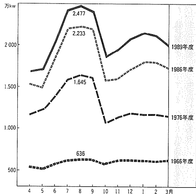
電気の使われ方(関西電力の場合) 月間最大電力年度別推移
